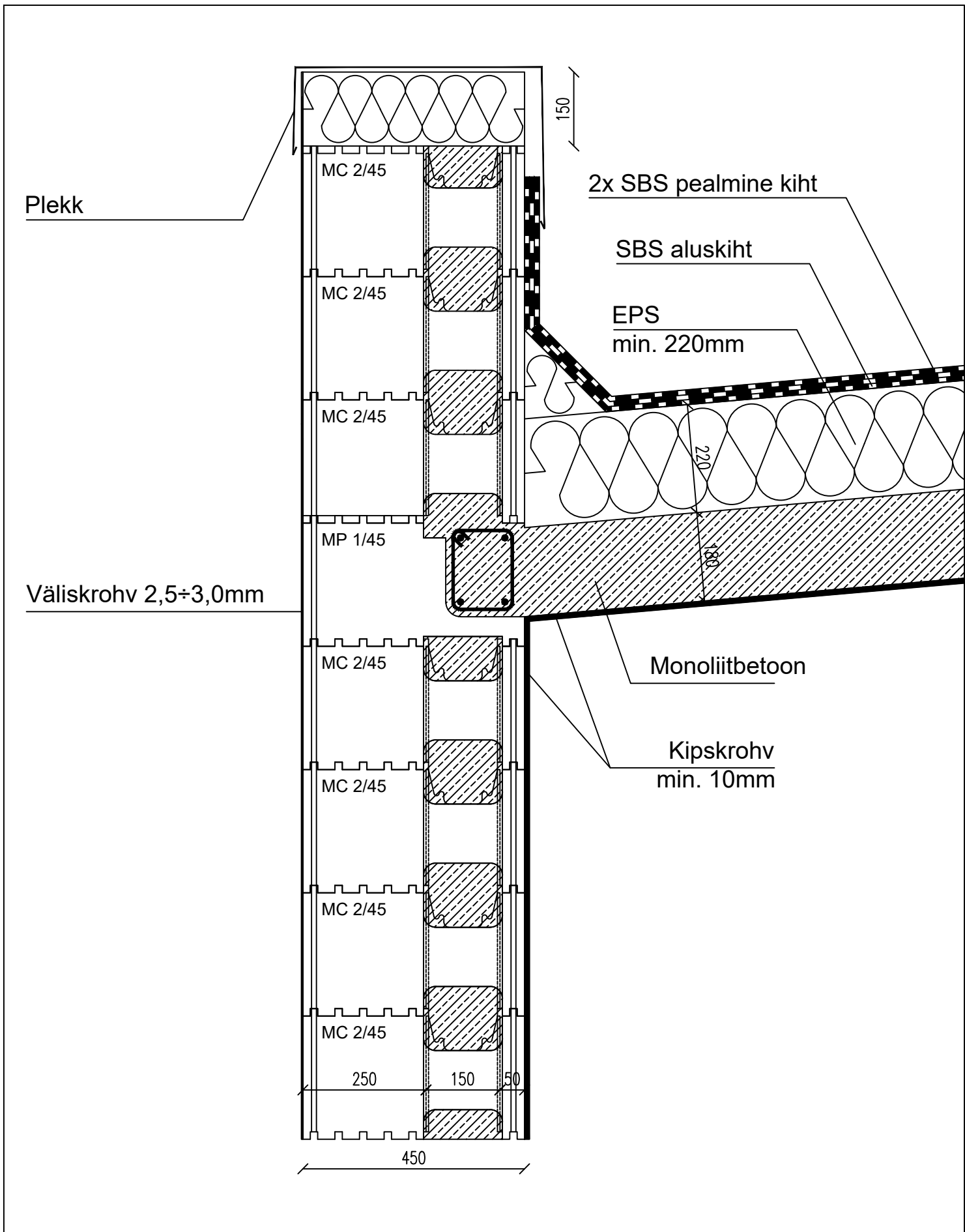
Lamekatuse ja seina sõlm
